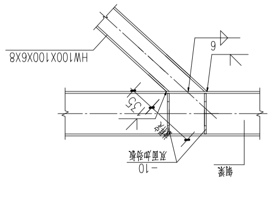
④ GC1与梁连接节点图
